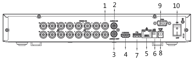
DH-XVR5116H-X
